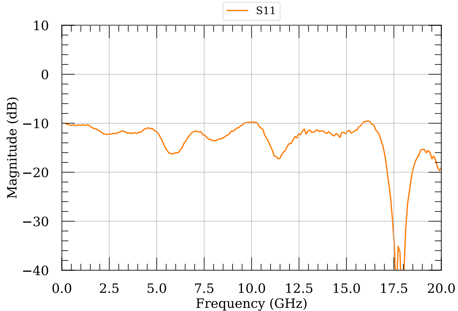
LNA S-params module066v2
